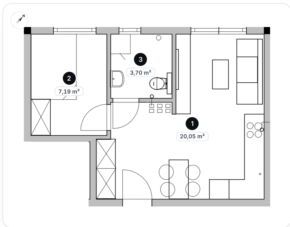
RZUT MIESZKANIA M31
