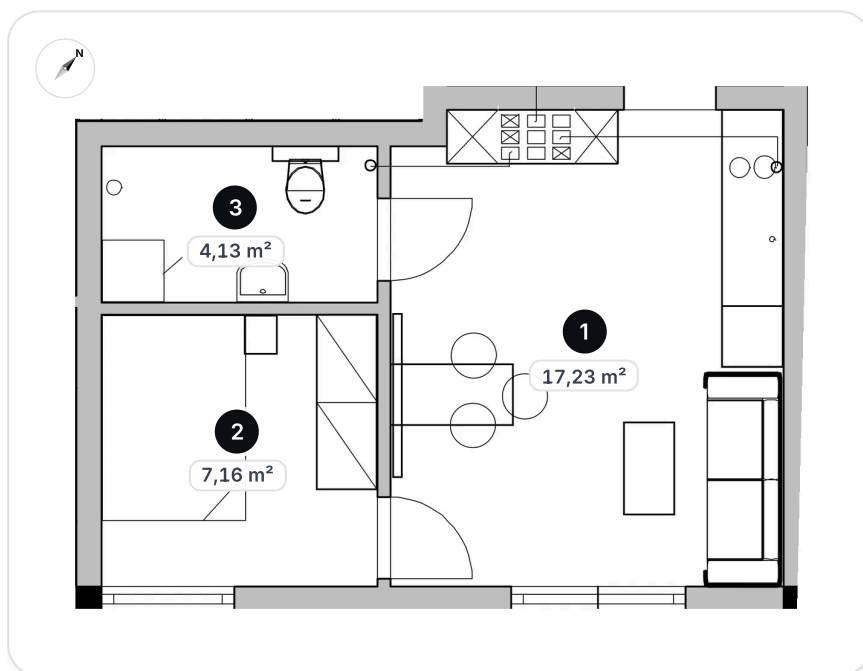
RZUT MIESZKANIA M10
