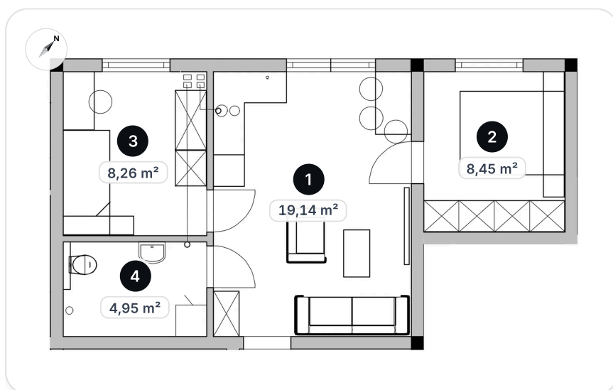
RZUT MIESZKANIA M12
