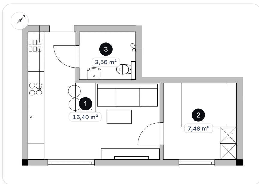
RZUT MIESZKANIA M15
