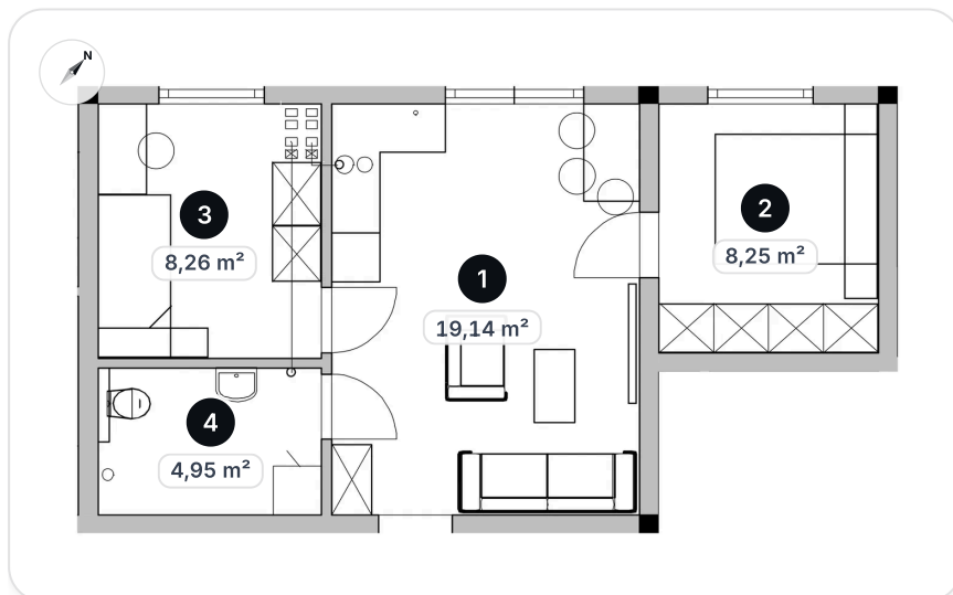
RZUT MIESZKANIA M18
