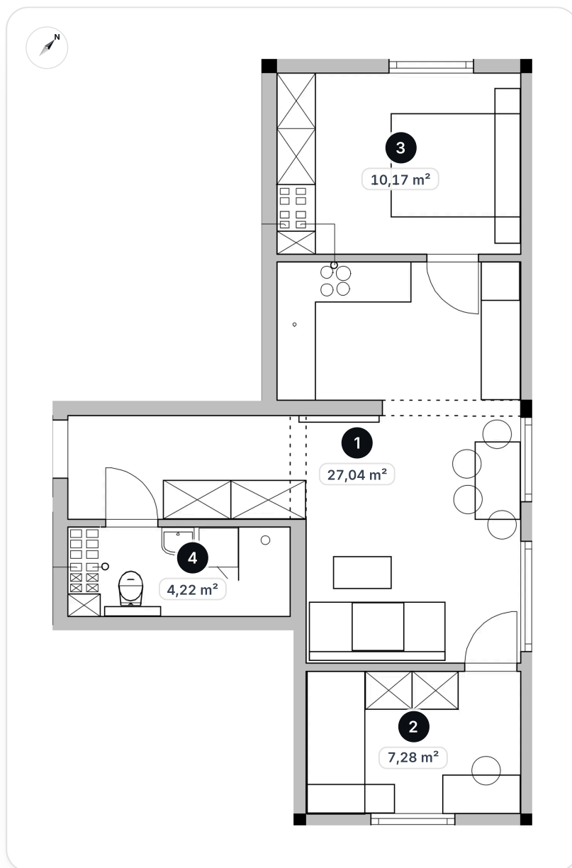
RZUT MIESZKANIA M20
