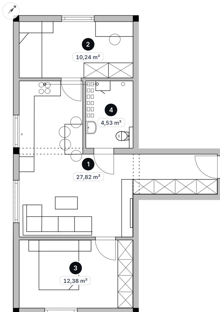
RZUT MIESZKANIA M35
