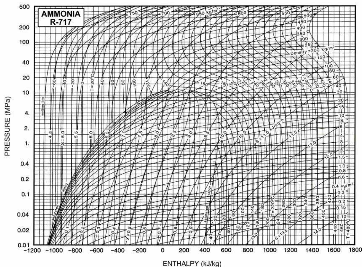
圖一 氨冷媒之壓焓圖
