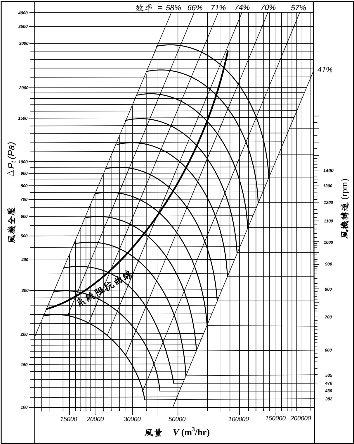
圖 2 風機型錄
