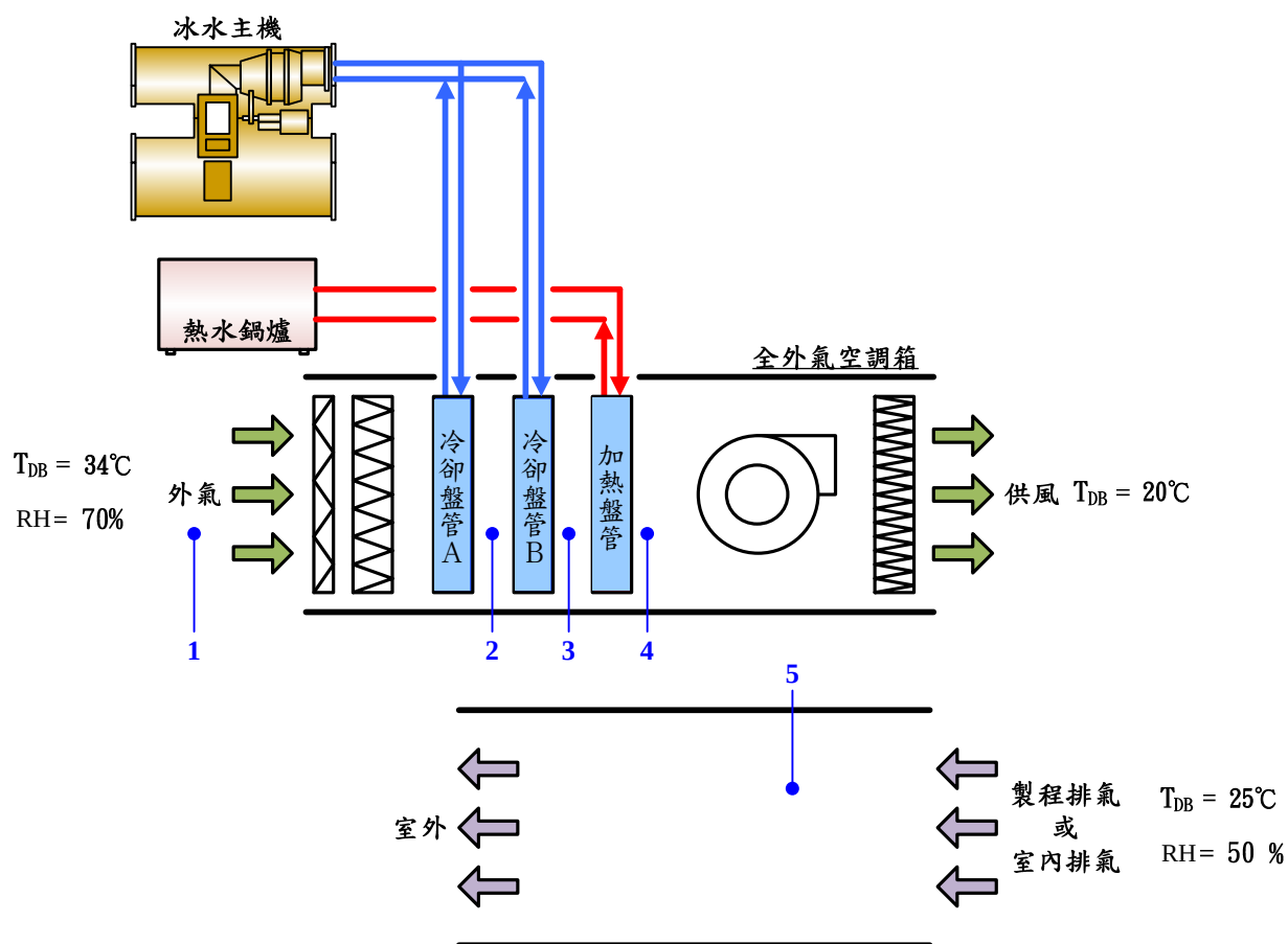
圖 3 全外氣空調箱示意圖
