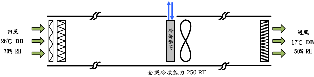
圖 1 空調系統示意圖
