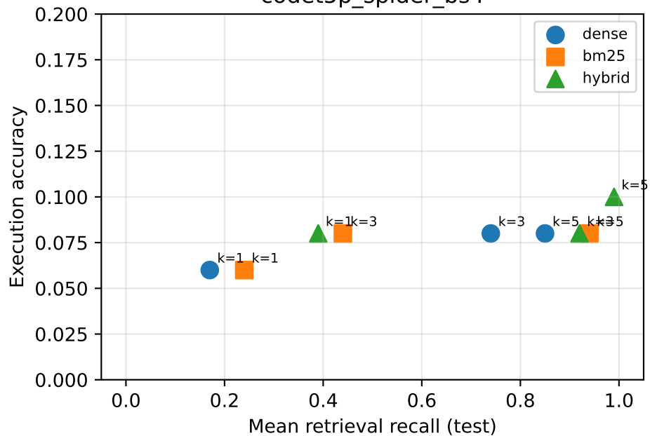
codet5p_spider_bs4
