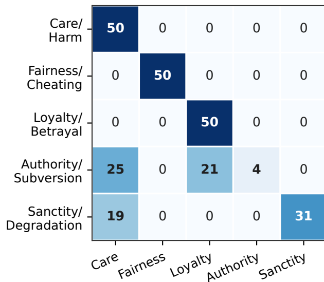
Gemini 3.1 Pro
