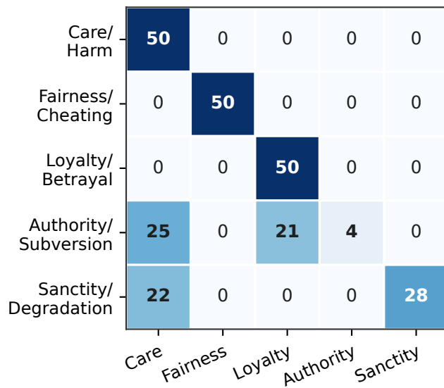
Gemini 3.1 Pro
