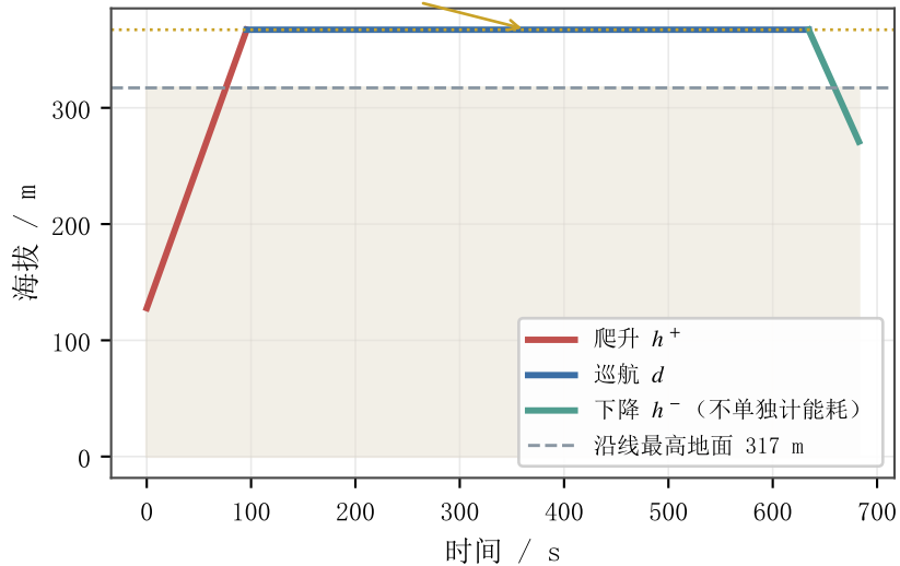
(a) 001巡航* $008最高飞行剖面(C 型, 最远航段)
