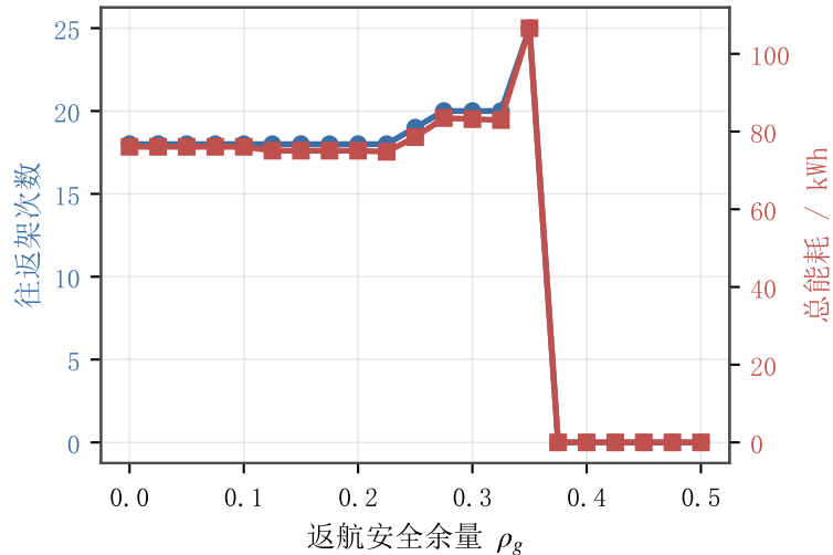
(b) \rho_g 是唯一强敏感参数 (架次 18→25)
