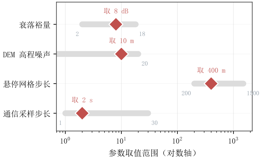
(a) 四类参数的取值范围与本文取值
