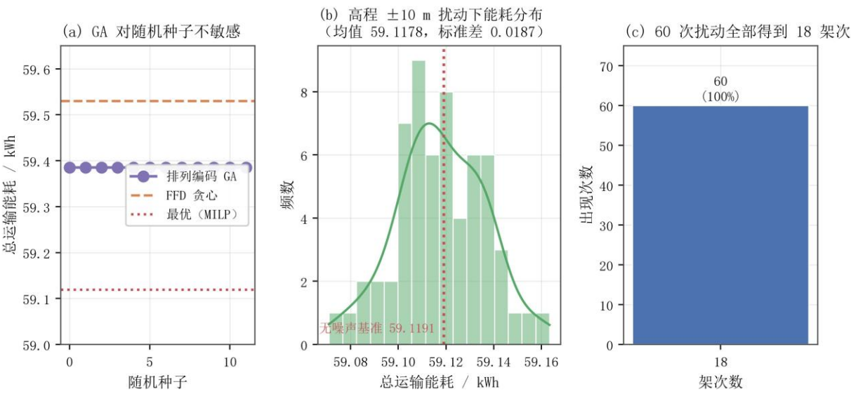
图 13.19 算法稳定性与地形数据蒙特卡洛
