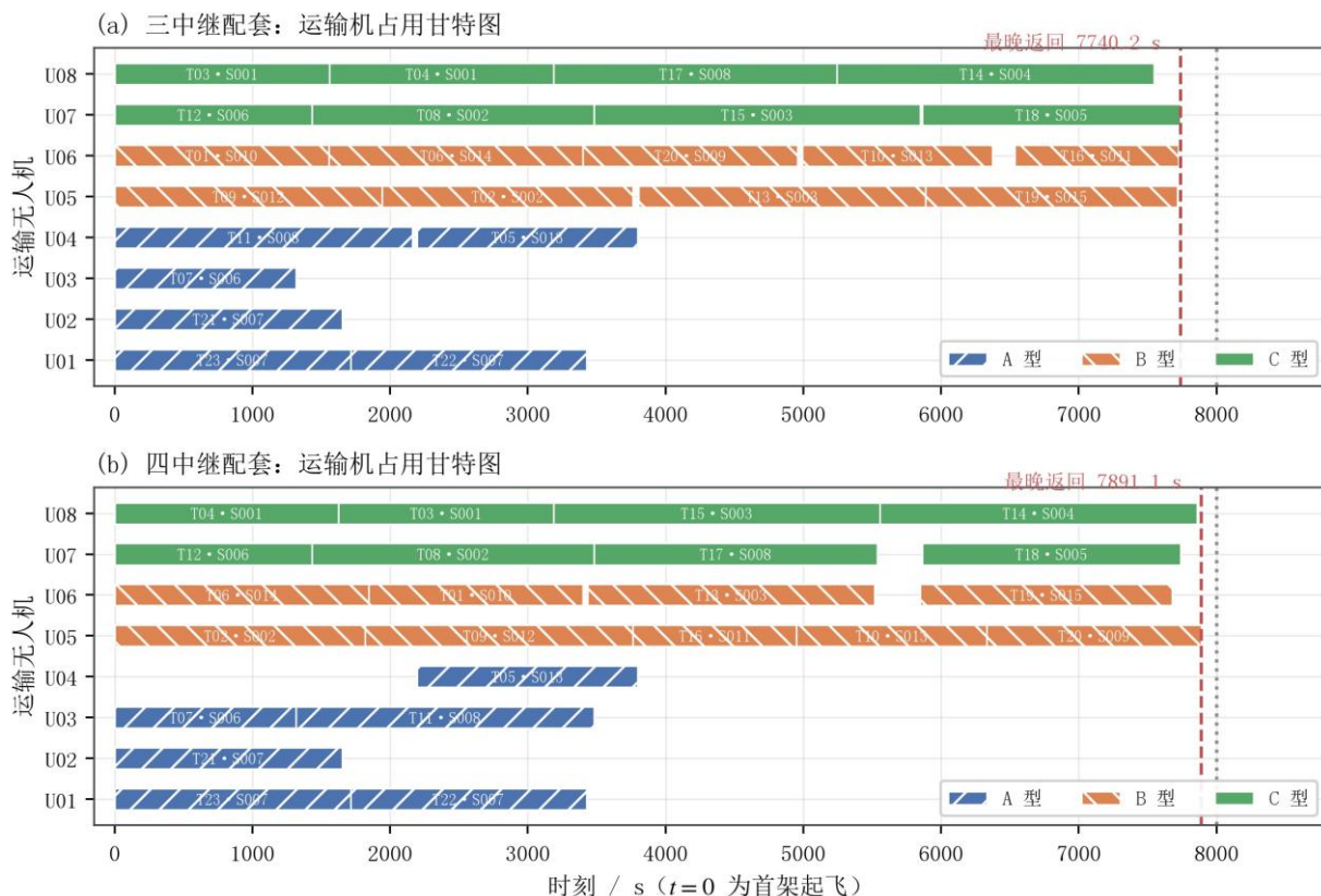
图 7.5 运输无人机占用甘特图
