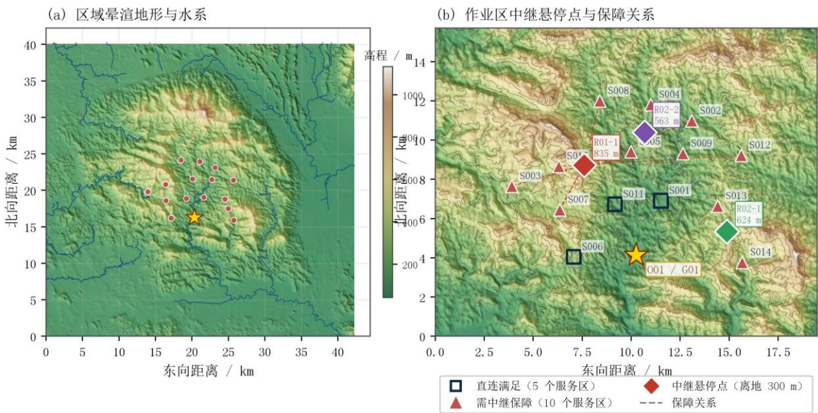
图 9.12 区域地形、中继悬停点与保障关系
