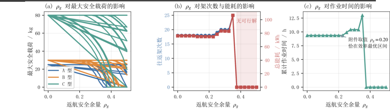
图 15 返航安全余量敏感性分析
