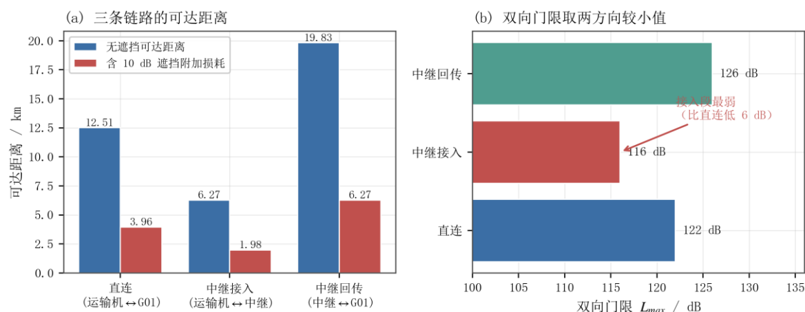
图 6 通信链路预算与双向门限
