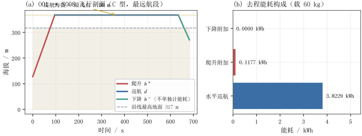
图 8 飞行剖面与去程能耗构成
