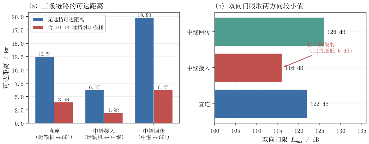
图 6 通信链路预算与双向门限
