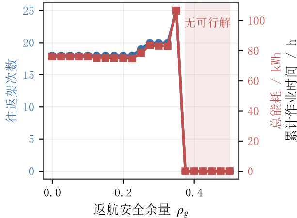
(b) \rho_g 对架次数与能耗的影响
