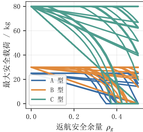
(a) \rho_g 对最大安全载荷的影响
