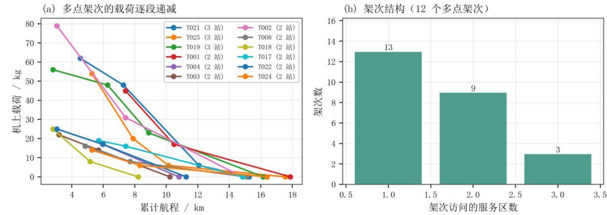
图 19 多点架次的载荷递减与架次结构
