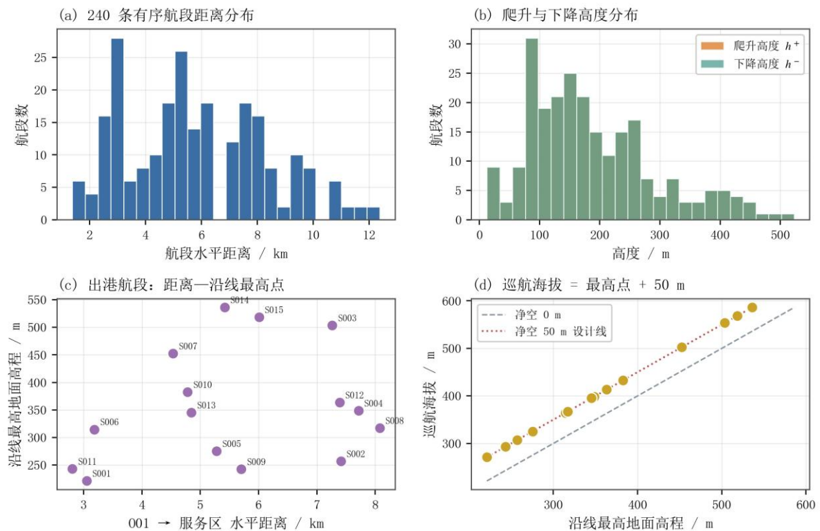
图 3 航段几何特征与巡航海拔确定规则
