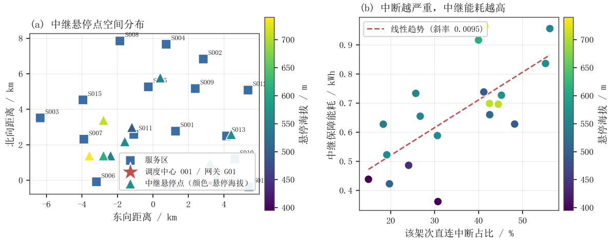
图 28 中继悬停点空间分布
