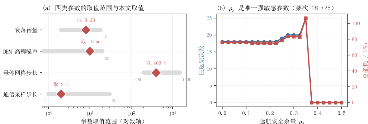
图 37 敏感性分析
