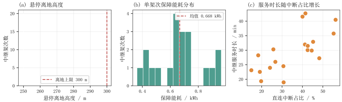
图 29 中继悬停参数与保障能耗
