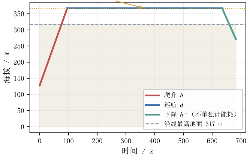
(a) 001巡航海拔008最高飞行剖面(C型, 最远航段)
