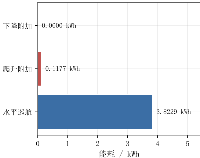
(b) 去程能耗构成 (载 60 kg)
