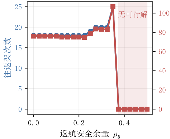
(b) \rho_g 对架次数与能耗的影响
