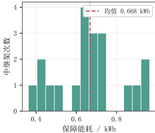
(b) 单架次保障能耗分布
