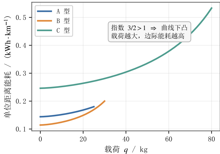
(b) 单位距离能耗随载荷上升 (凸性)
