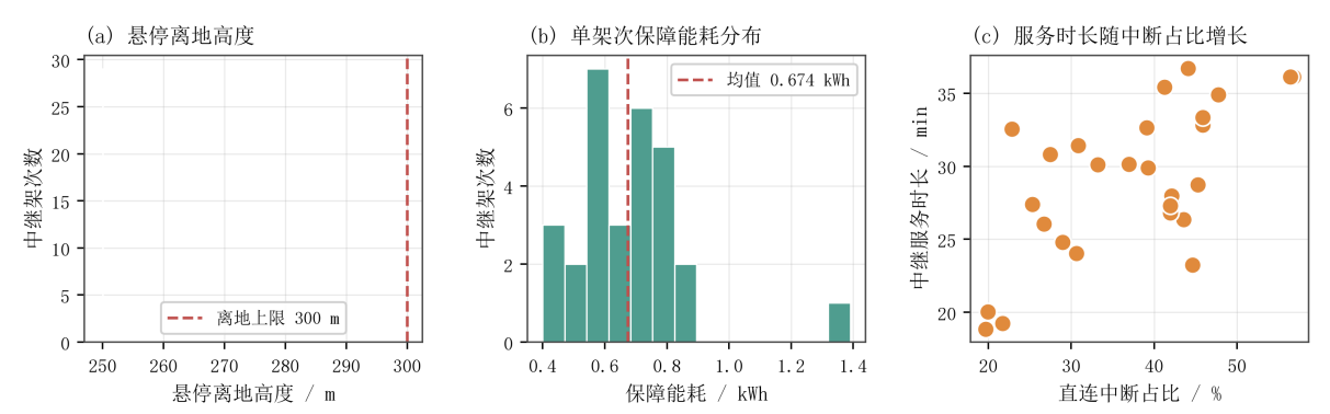
图 29 中继悬停参数与保障能耗
