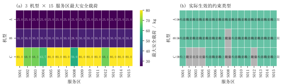
图 10 最大安全载荷热力图与生效约束
