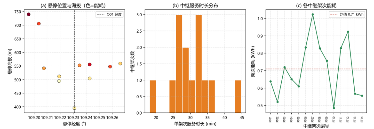
图 18 中继选址特征
