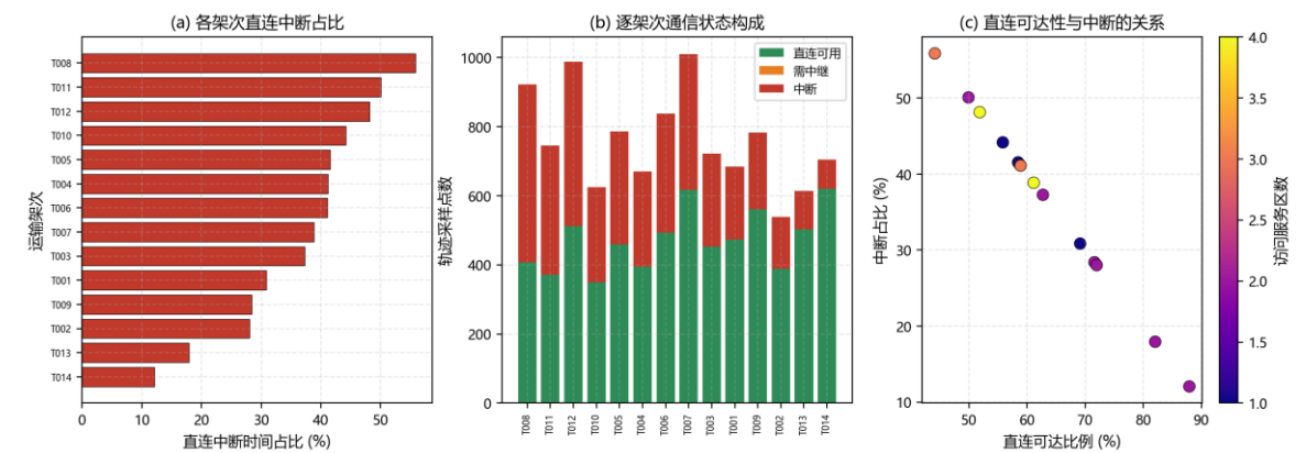
图 16 连续通信诊断（轨迹逐时刻采样）
