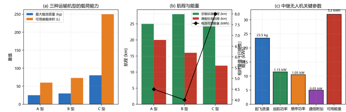
图 5 机型与中继参数一览
