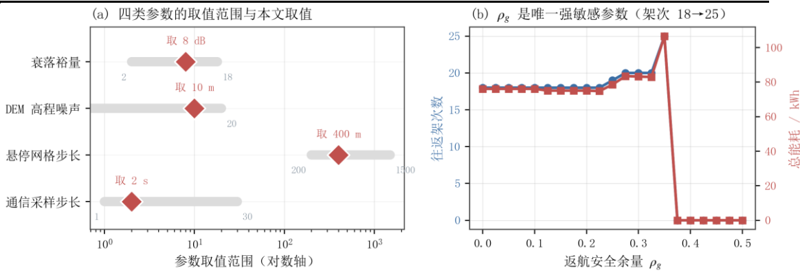
图 37 敏感性分析
