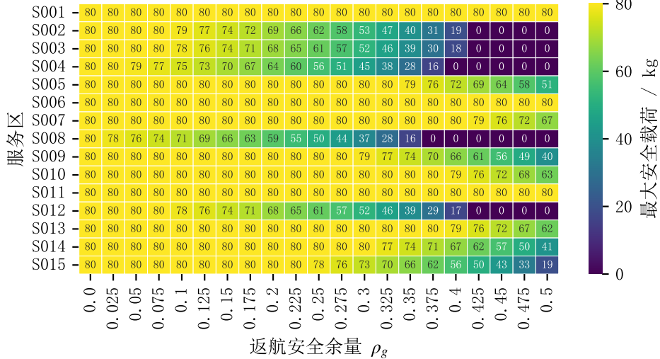
(a) C 型最大安全载荷随 \rho_g 的演化
