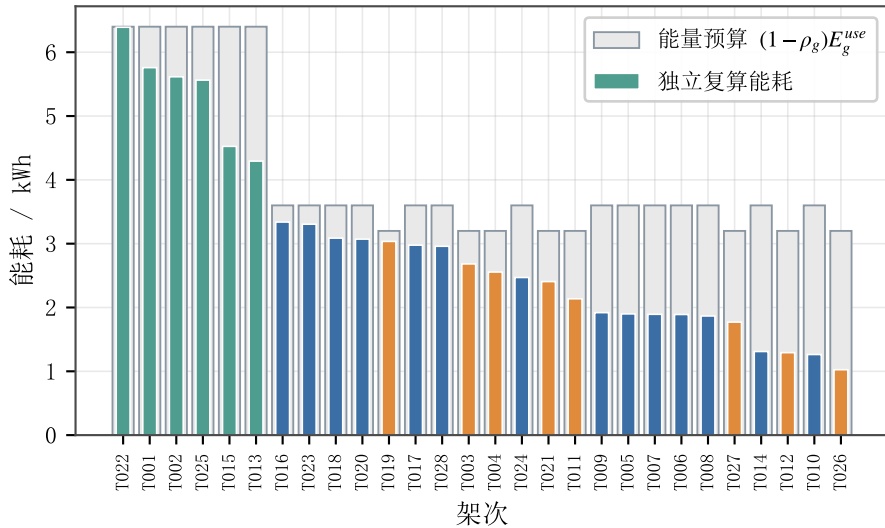
(a) 逐架次能耗与能量预算（全部在预算内）
