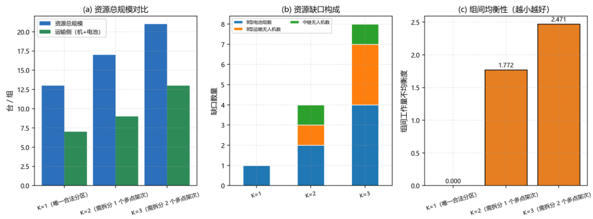
图 21 分区方案多指标对比
