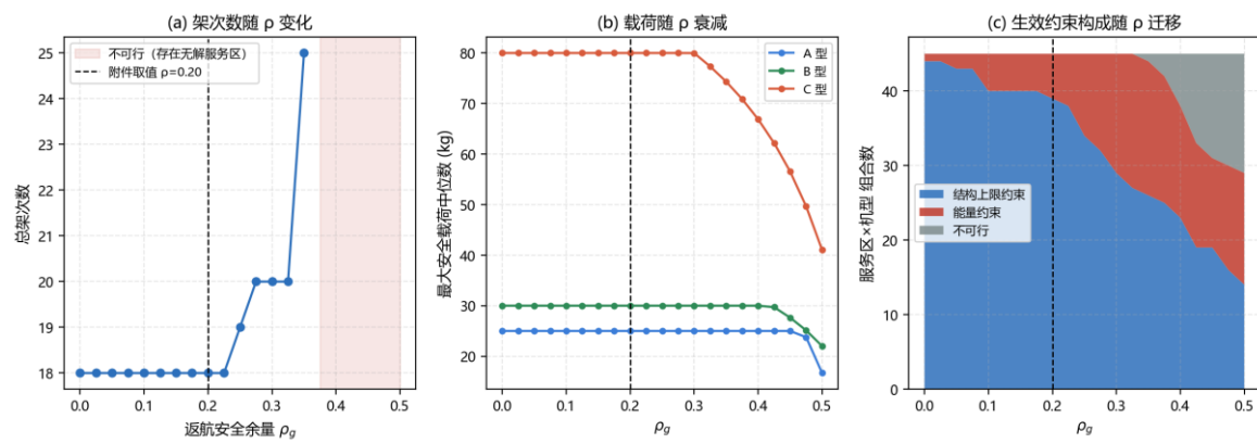
图 12 返航安全余量 ho_g 敏感性分析
