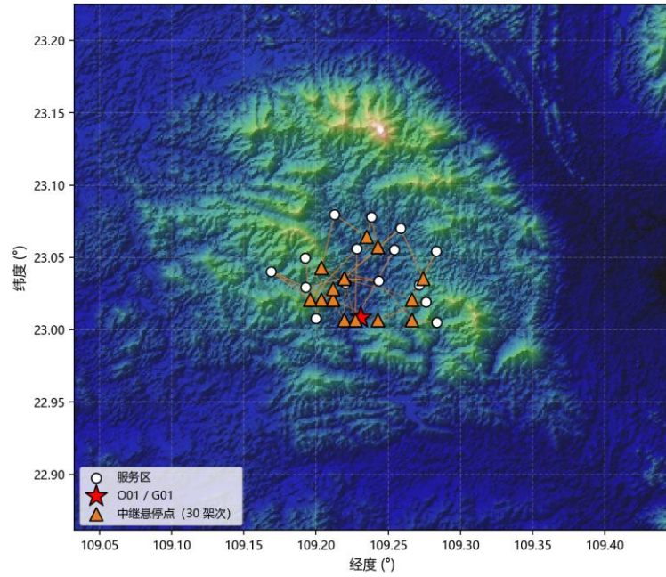
图 17 中继悬停点与通信保障关系
