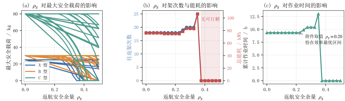
图 15 返航安全余量敏感性分析
