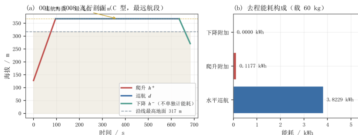
图 8 飞行剖面与去程能耗构成
