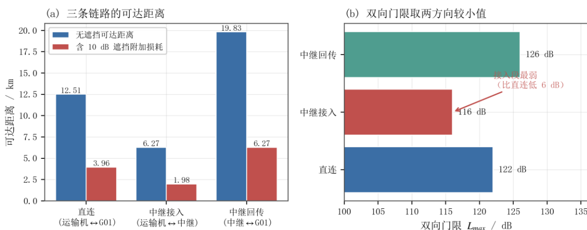
图 6 通信链路预算与双向门限
