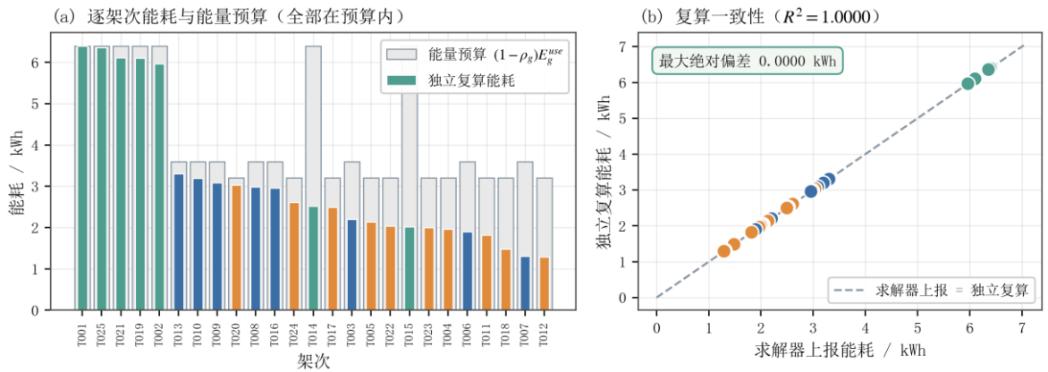
逐架次能耗与能量预算对比
