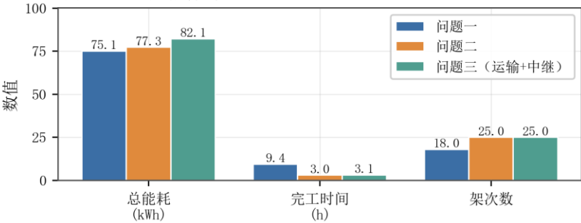
(d) 四问主要指标对比
