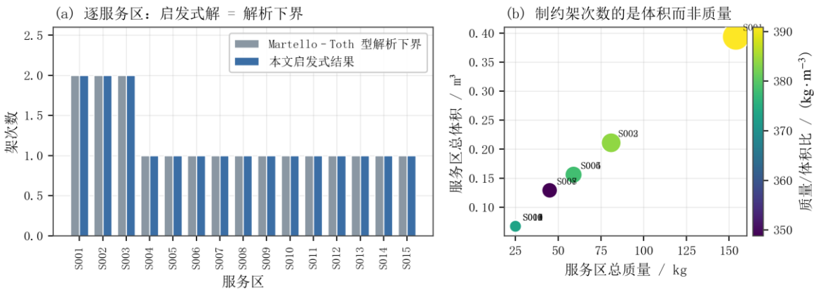
逐服务区架次数下界与启发式差距
