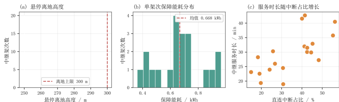
中继悬停参数与保障能耗
