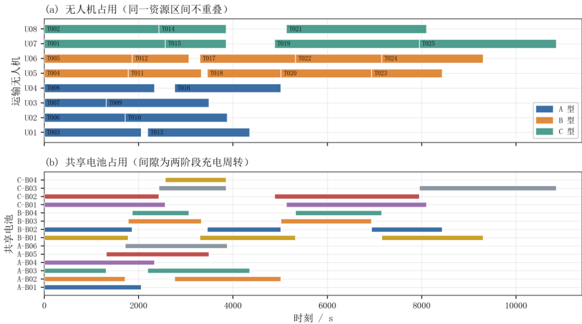
无人机与共享电池的占用时序
