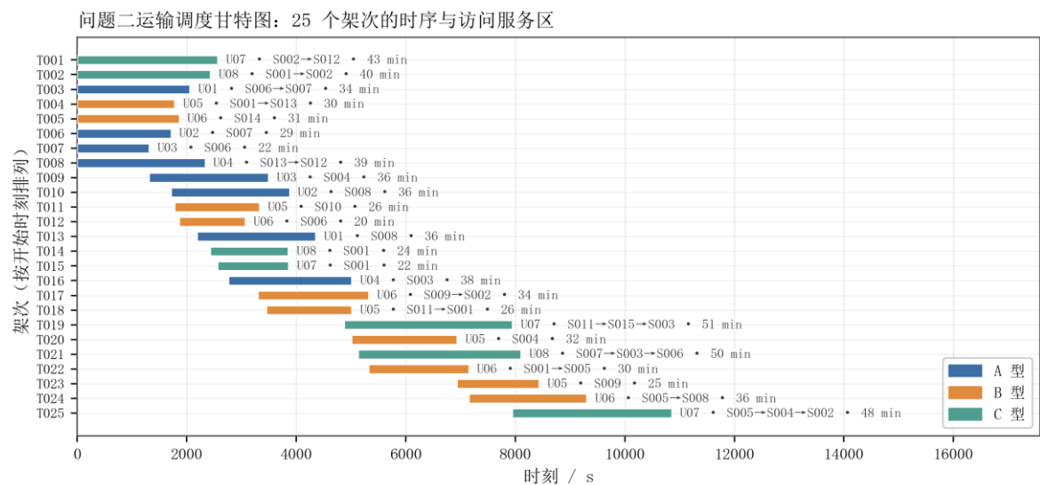
运输调度甘特图
