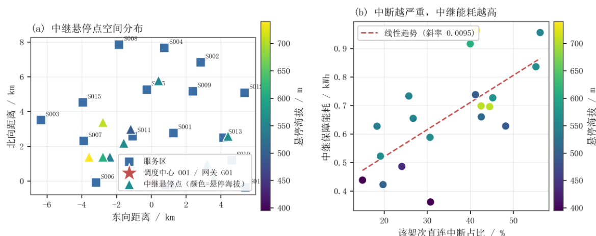
中继悬停点空间分布
