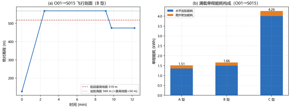
图 7 飞行剖面与能耗构成
