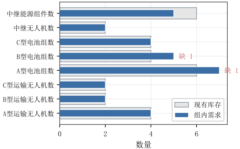
(b) K=1 缺口: 1 组A型电池、1 组B型电池
