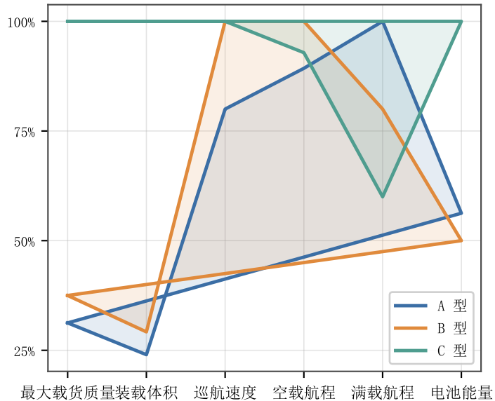
(a) 三种机型能力归一化对比
