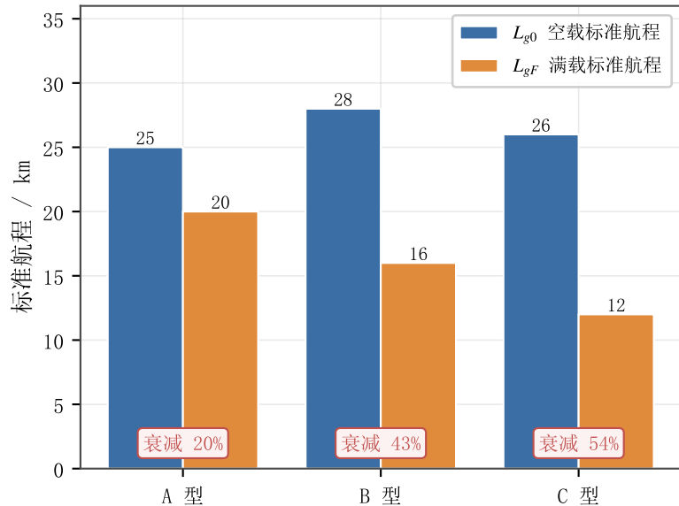
(b) 空载 / 满载标准航程差距
