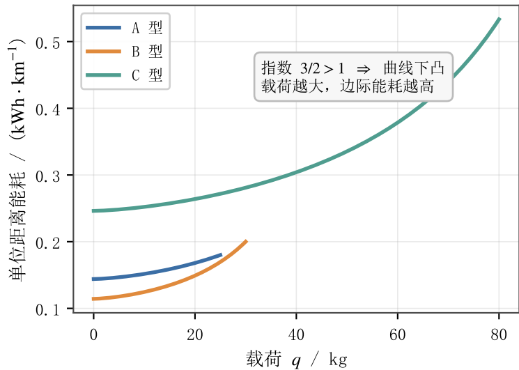
(b) 单位距离能耗随载荷上升（凸性）
