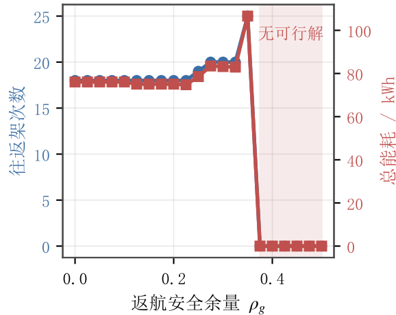
(b) \rho_g 对架次数与能耗的影响
