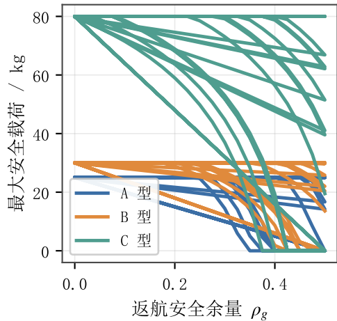
(a) \rho_g 对最大安全载荷的影响
