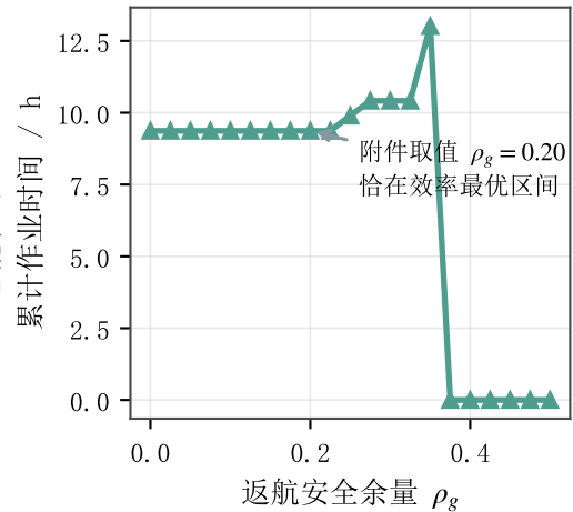
(c) \rho_g 对作业时间的影响
