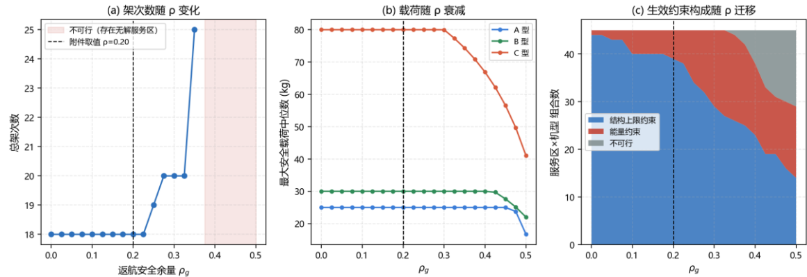
图 12 返航安全余量 \rho_g 敏感性分析
