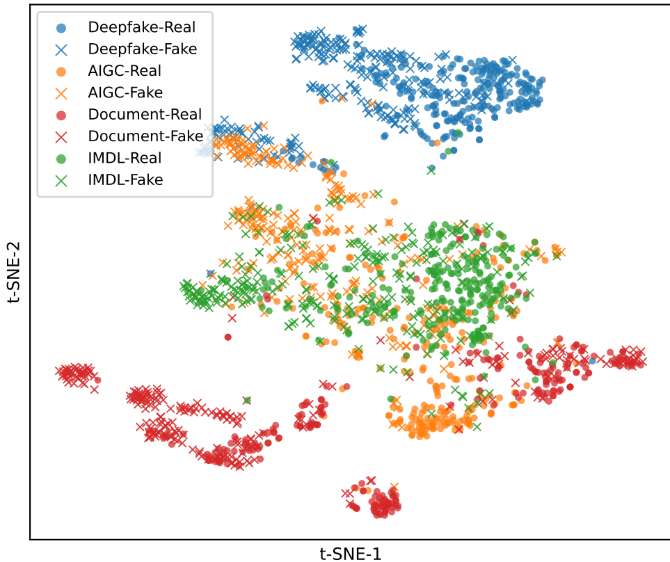
(b) DINO-FFT
