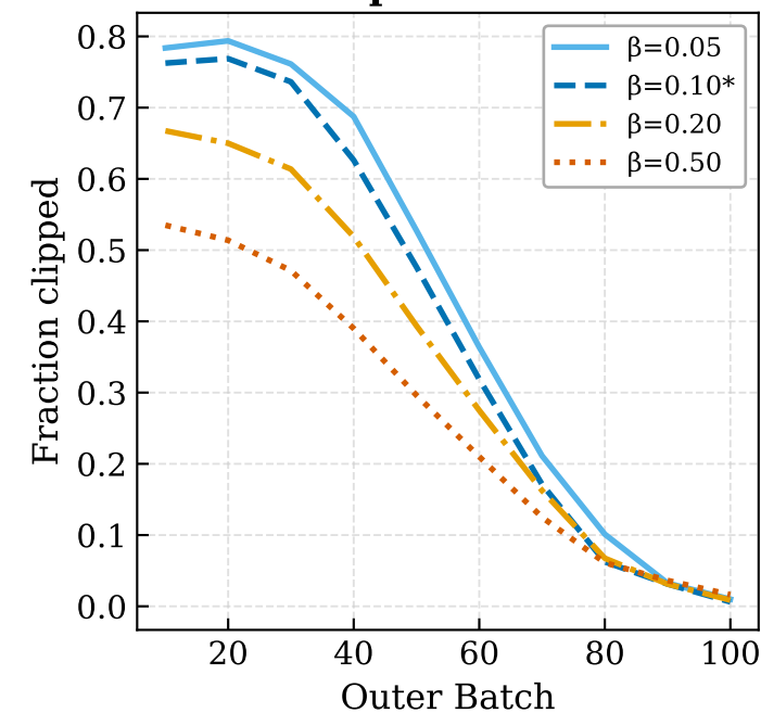
Clip Fraction
