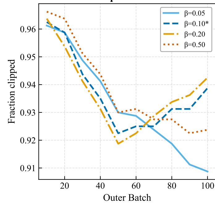
Clip Fraction
