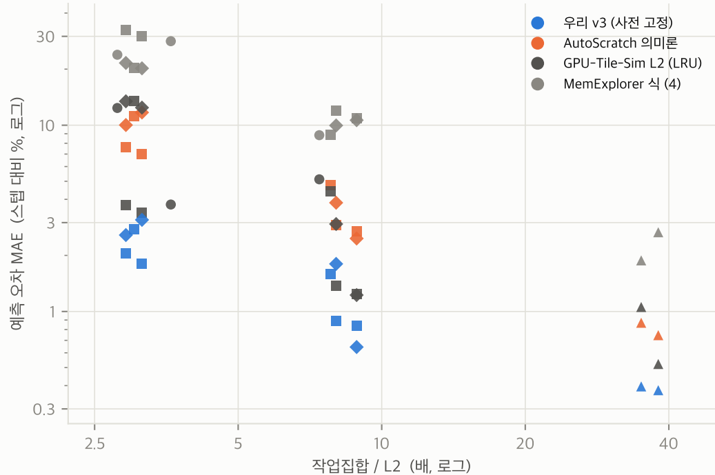
(b) 예측기 사이의 차이는 작업집합이 L2 에 가까울 때만 크다
