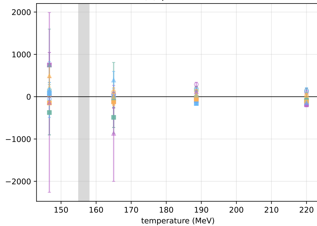
SU(2)spinxchiral X-A
