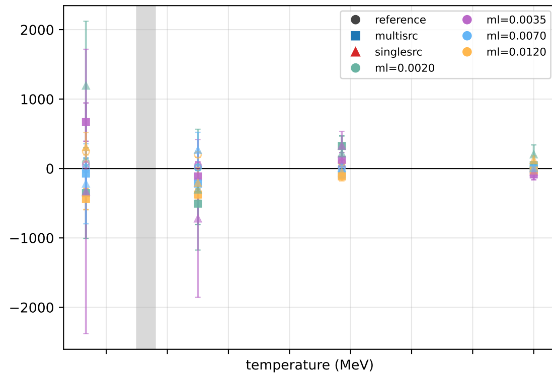
SU(2)spinxchiral X-A
