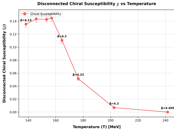
(a) No-RM 磁化率 (对标 sucep_calc.py 标准红系配色)
