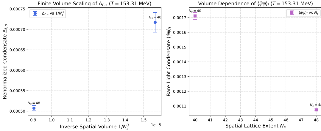
图 5: 固定温度 T = 153.31 MeV 下有限空间体积标度外推图。左图为重整化凝聚 \Delta_{l,s} 随逆体积 1/N_s^3 演化; 右图为裸光夸克凝聚随 N_s 的关系。
