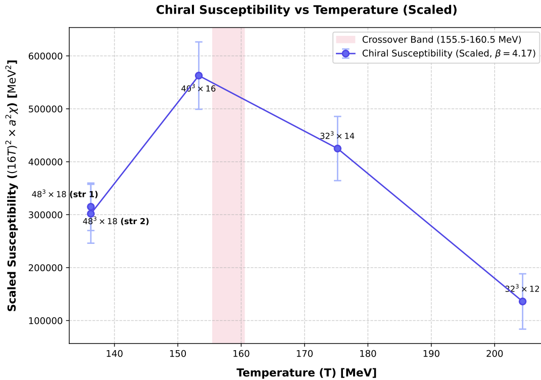
图 8: 有限时间延展标度系综 ( \beta = 4.17, m_\ell = 0.0020, m_s = 0.0400 ) 连续标度手征磁化率 (16T)^2 a^2 \chi [MeV 2 ] 随温度演化图谱。
