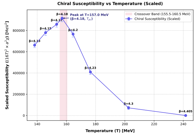
(b) 连续标度 RM 磁化率 (对标 plot_chisce.py 靛蓝配色)
