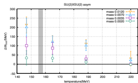
SU(2)_L \times SU(2)_R (V-AV)
