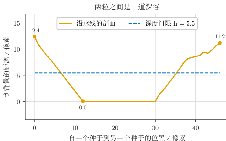
图 9: 为什么看深度而不看距离。左为粘连块的距离变换，右为沿两个种子连线的剖面，虚线是 h-maxima 的深度门限。
