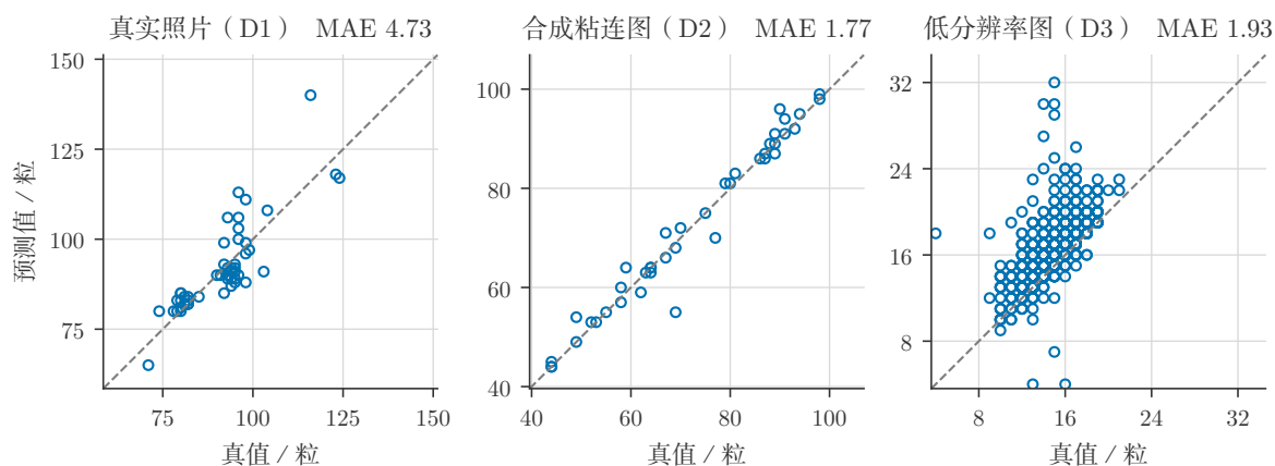
图 13: 预测值与真值对照, 虚线表示两者相等。
