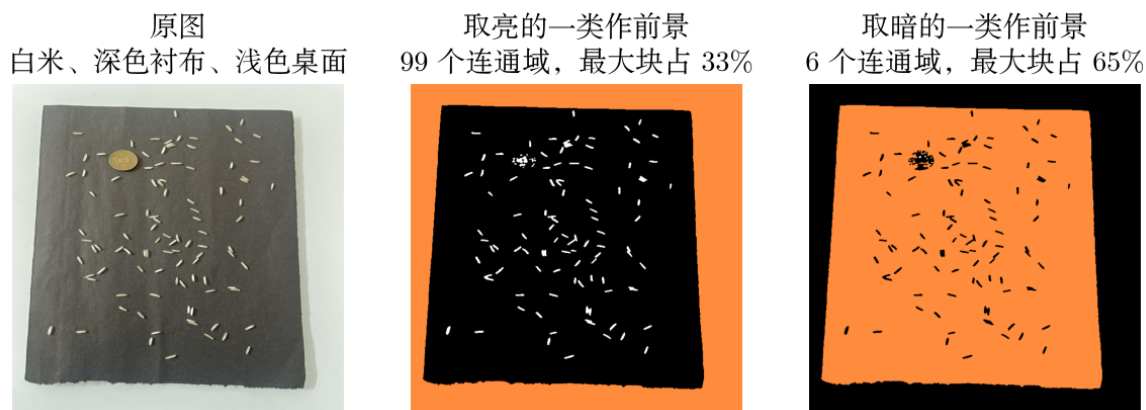
图 6: 固定用灰度两类阈值的后果, 橙色为该二值图中最大的连通域。前景取亮或取暗都会多出一片巨大的伪前景。
