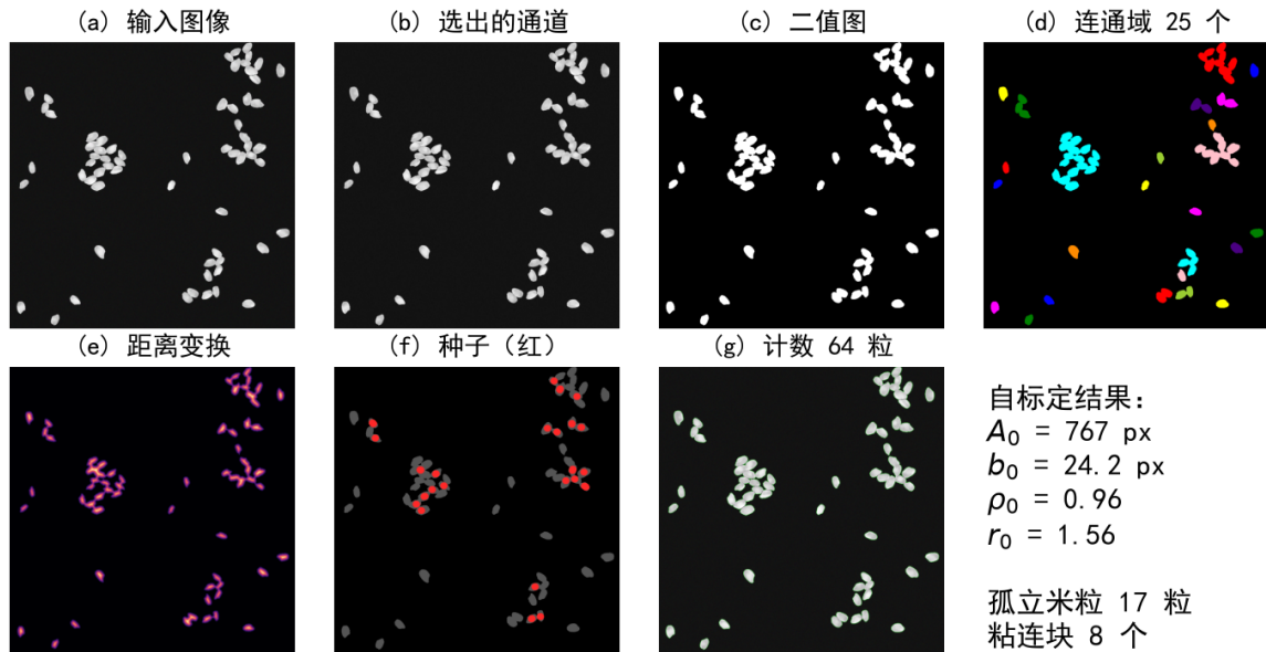
图 3: 各步骤在一张合成图上的中间结果。
