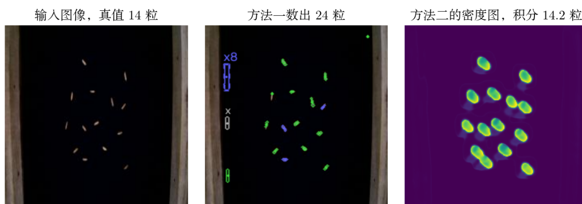
图 18: 同一张低分辨率图上两种方法的对照。中图里左侧的虚线框是方法一把木框亮边当作粘连块后按面积折算的 8 粒, 右图为学生模型预测的密度图。
