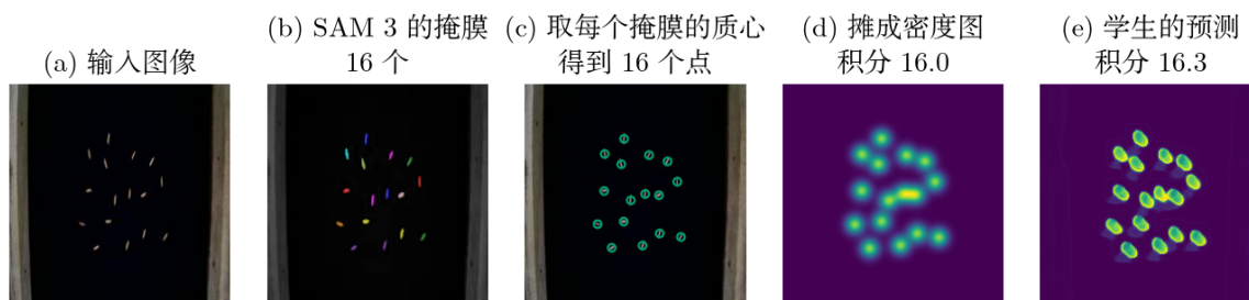
图 17: 方法二的流程。教师给出掩膜，取质心得到点标签，每个点摊成一个高斯就是训练目标，学生学着把这张密度图预测出来，其积分即为粒数。
