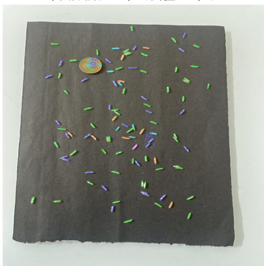
图 20: 真实照片 D1 场景一，左为本文方法、右为 SAM 3。
