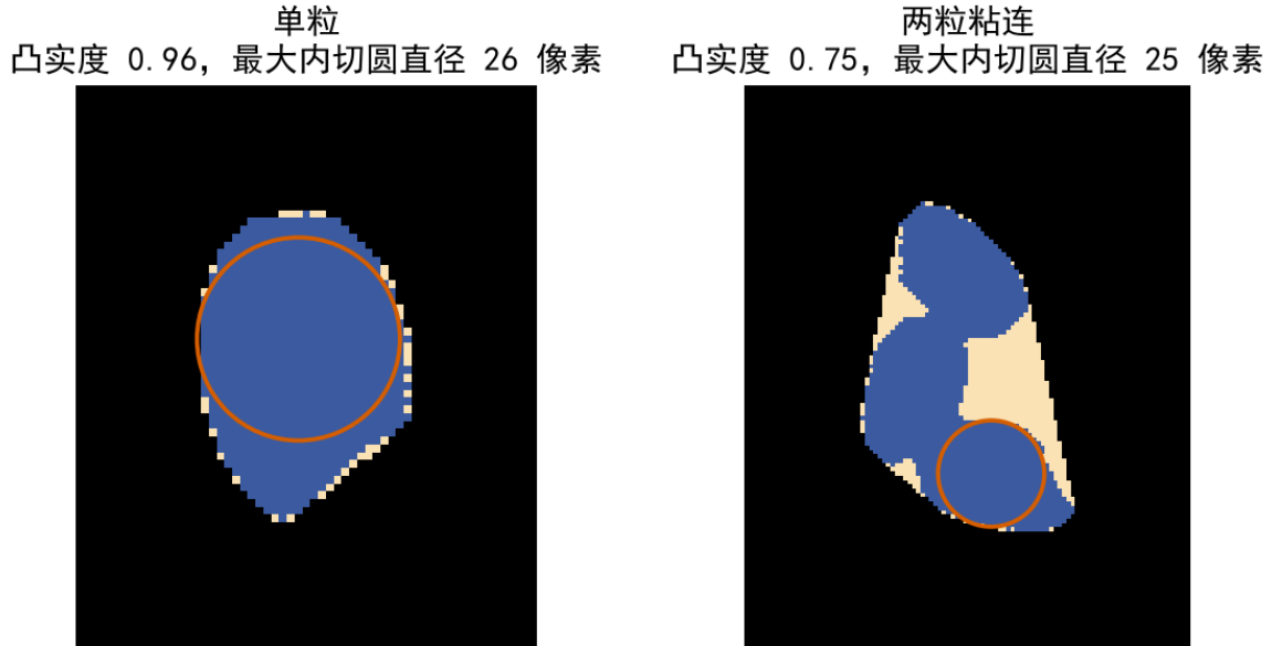
图 7: 单粒与粘连块的对照。蓝色为区域本身, 浅色为凸包多出的部分, 橙圈为最大内切圆。
