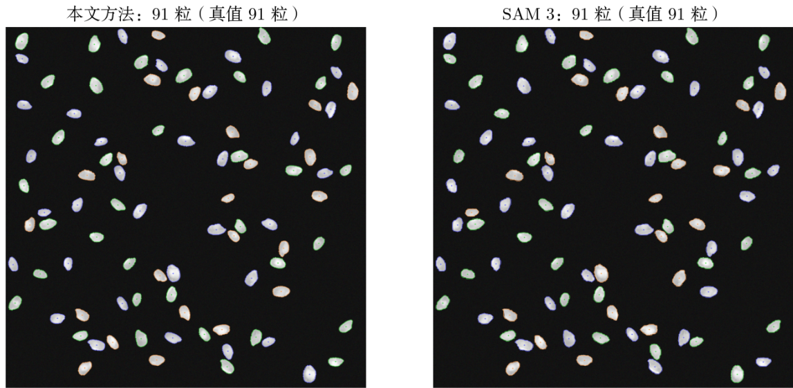
图 19: 合成粘连图 D2 中不粘连的场景，左为本文方法、右为 SAM 3。
