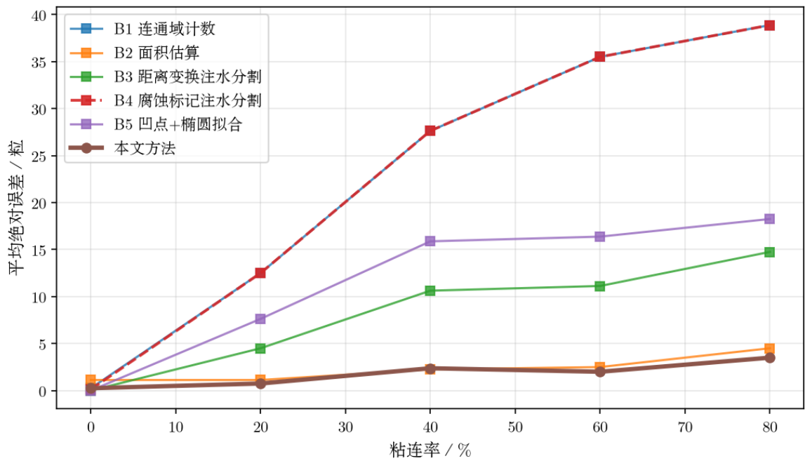
图 11: 计数误差随粘连率的变化。
