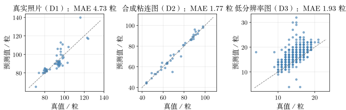
图 12: 预测值与真值对照, 虚线表示两者相等。
