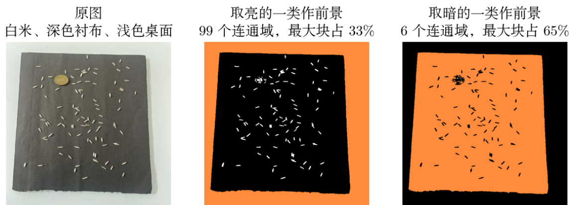
图 5: 固定用灰度两类阈值的后果，橙色为该二值图中最大的连通域。前景取亮或取暗都会多出一片巨大的伪前景。
